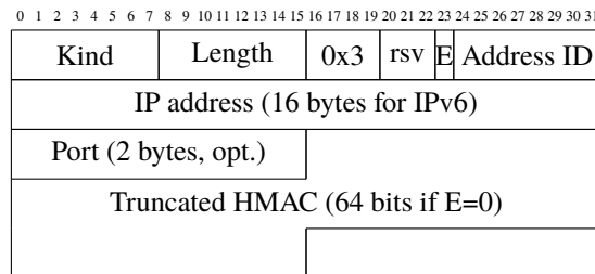
Fig. 3.37: The MP_PRIO option
