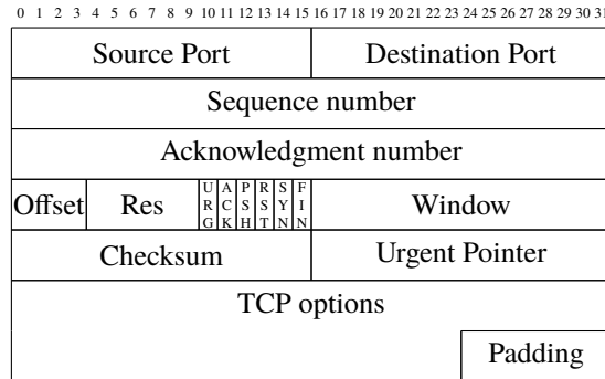
Fig. 3.32: The TCP header
