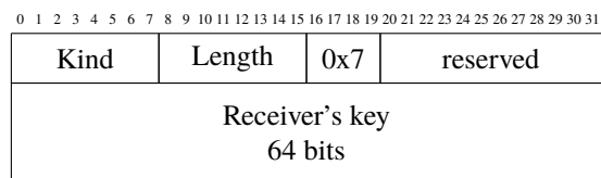
Fig. 3.44: The MP_TCPRST option
